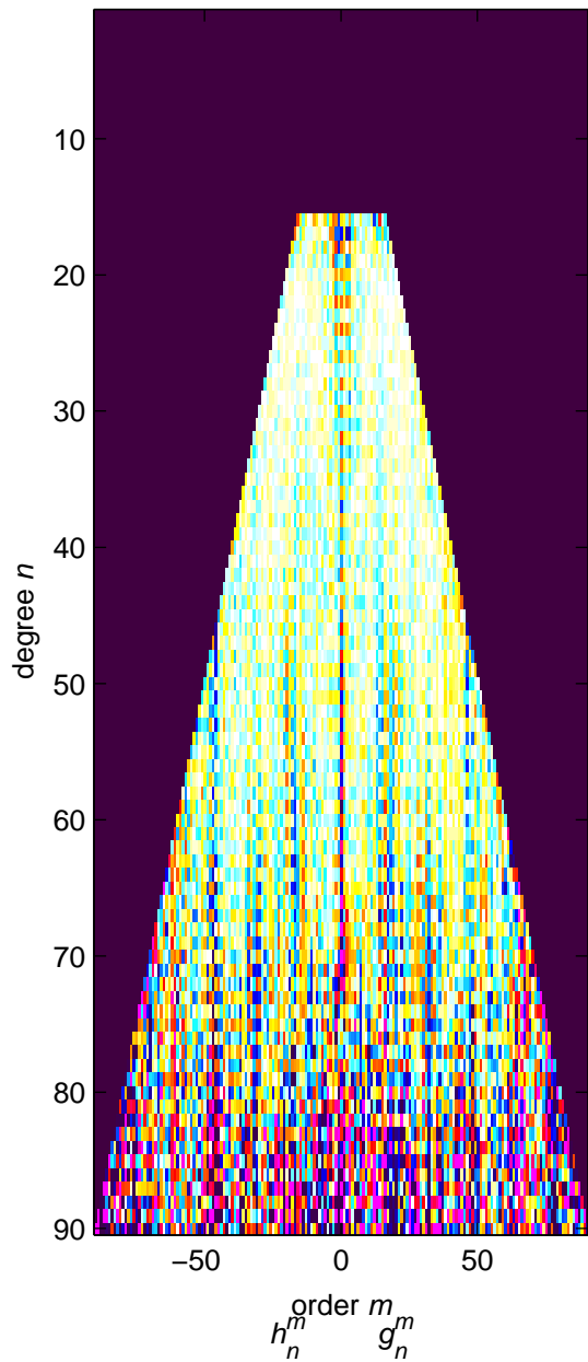
CI - CHAOS-6
