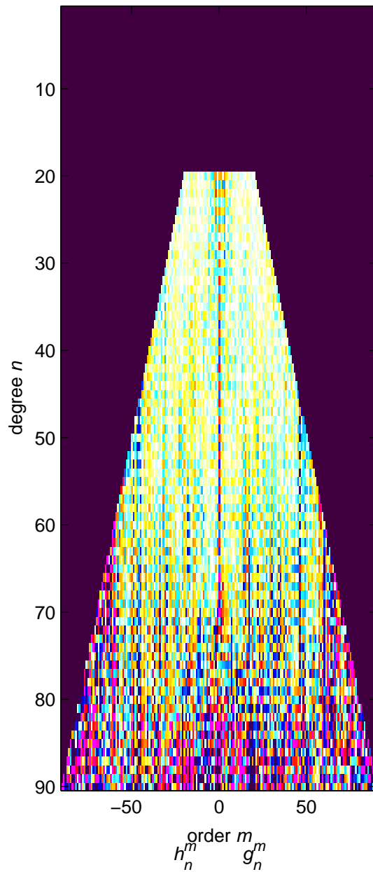
CI - MF7
