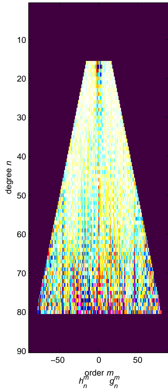
CI - SIFM+
