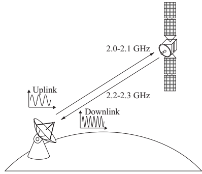
b S-band Doppler
