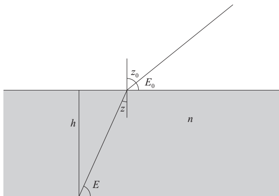
Fig. 6.12. Atmospheric refraction
